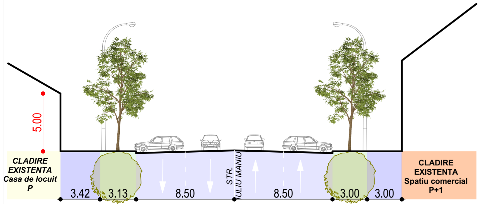
SECTIUNE STRADA IULIU MANIU - SITUATIE EXISTENTA
