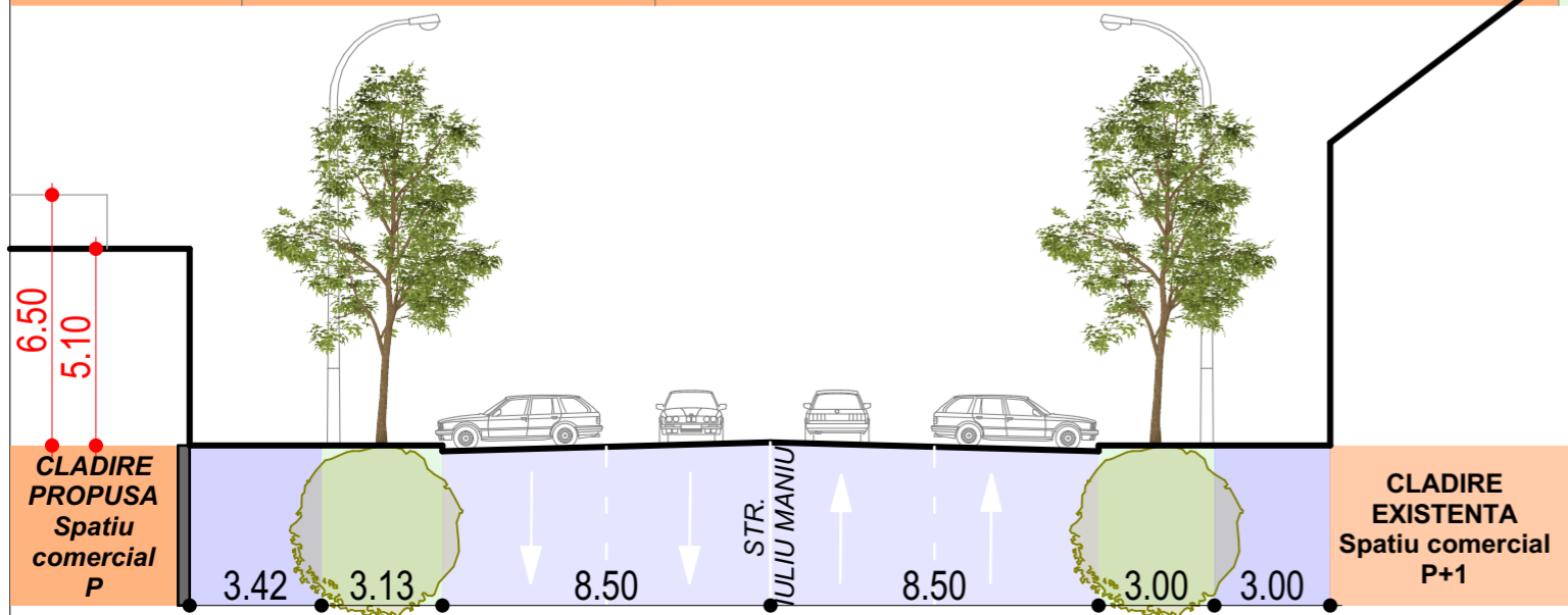
SECTIUNE STRADA IULIU MANIU - SITUATIE PROPUA
